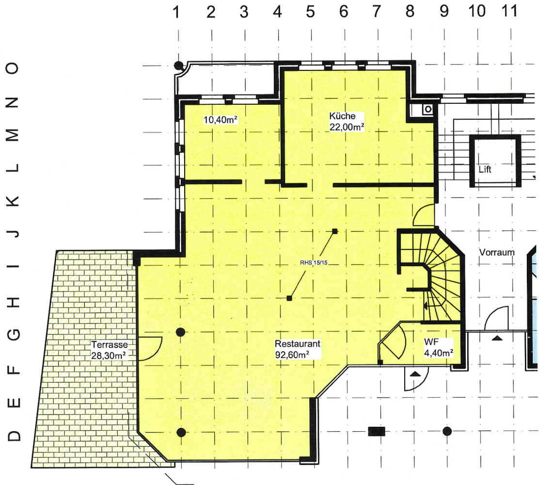
Grundriss Erdgeschoss
